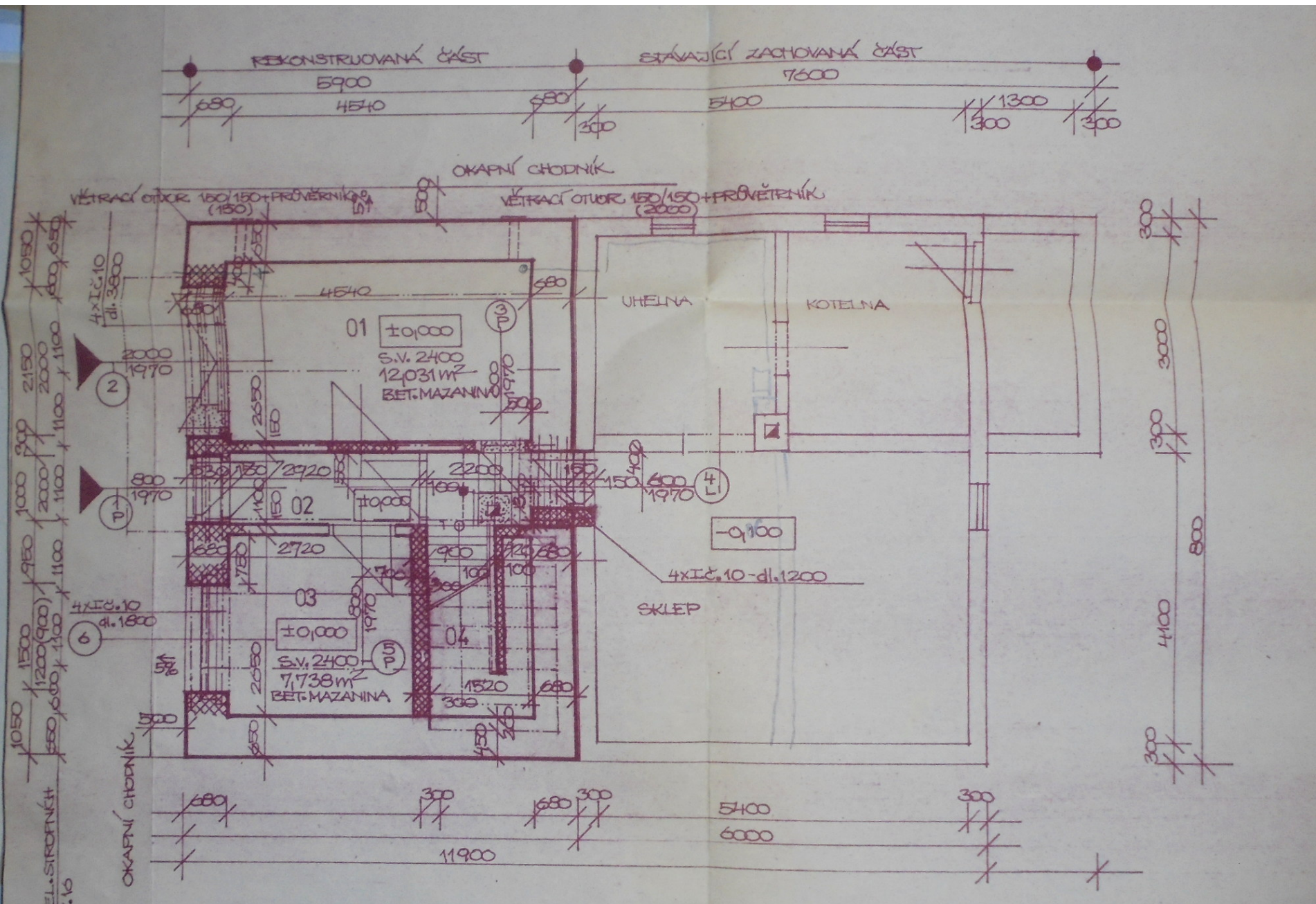
PŮDORYS 1. podlaží m1:50
